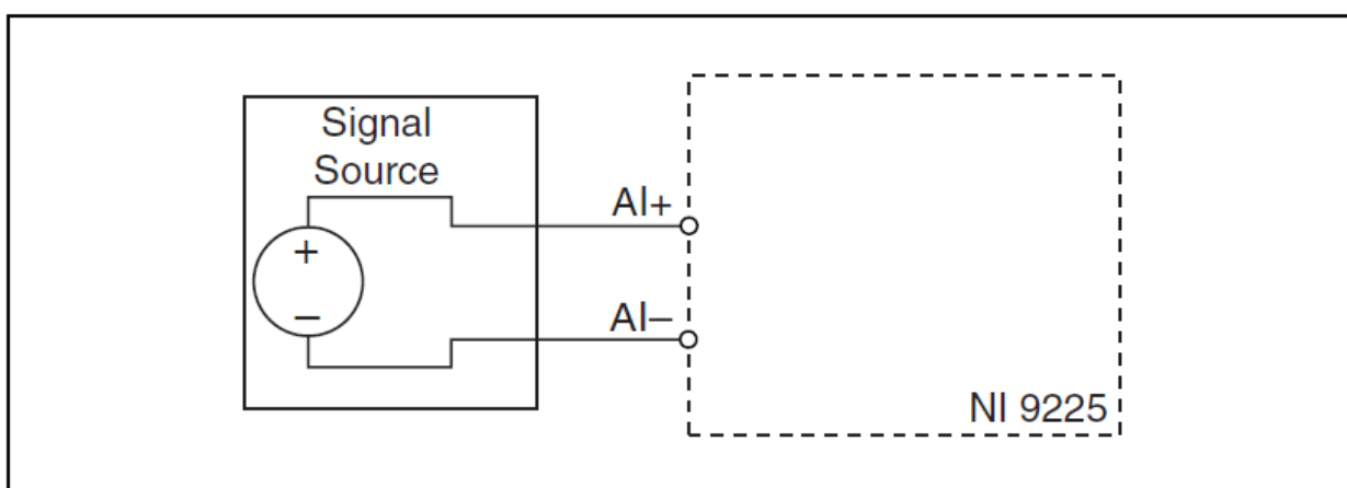
Рисунок 4. Подключение плавающего сигнала к NI 9225
