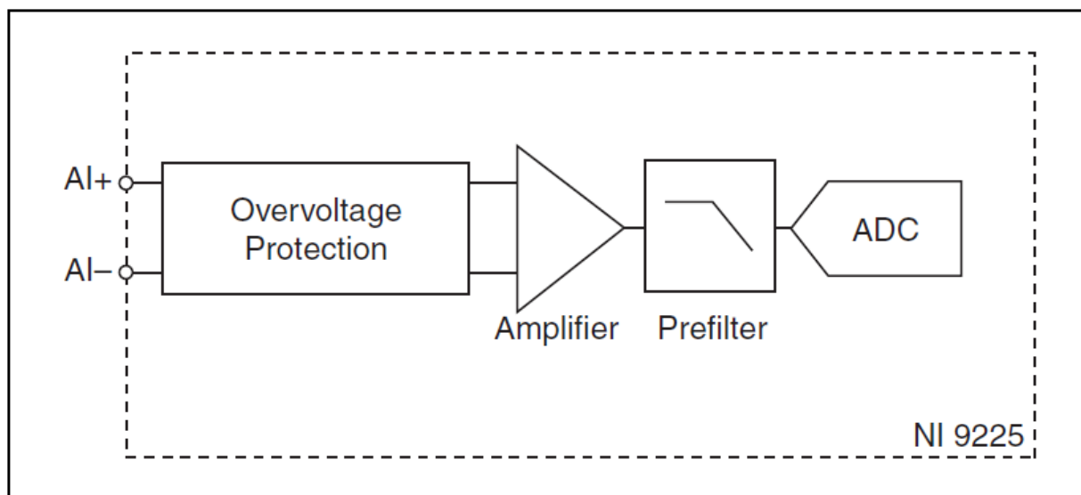
Рисунок 5. Электрическая схема входного канала NI 9225.
