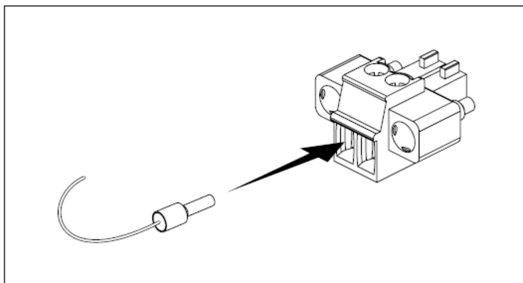
Рисунок 6. 2-разъемный разборный винтовой терминал для подключения с обжимкой.
