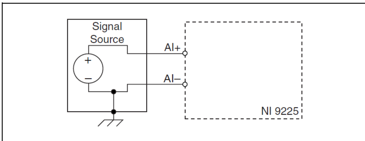
Рисунок 3. Подключение заземленного сигнала к NI 9225
