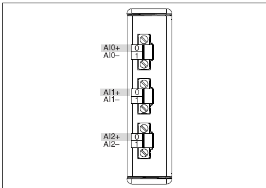
Рисунок 2.. Назначение выводов в NI 9225
