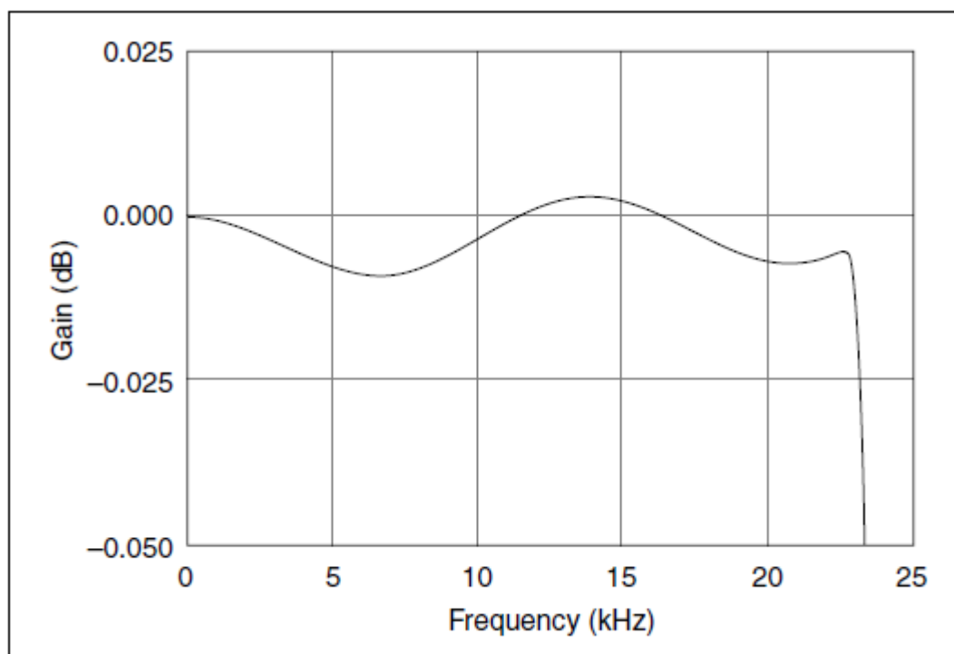
Рисунок 7. Типовая неоднородность полосы пропускания NI 9225.
