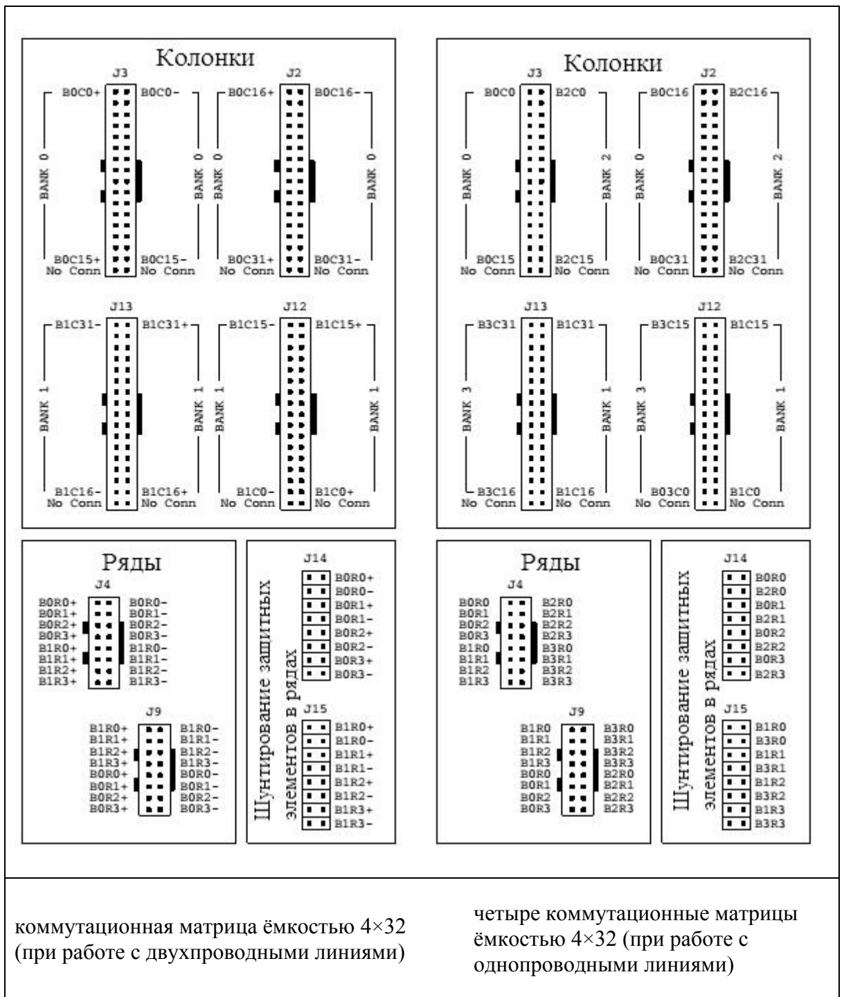
Рисунок 2. Цоколёвка соединителей терминального блока NI TB-2646B.
